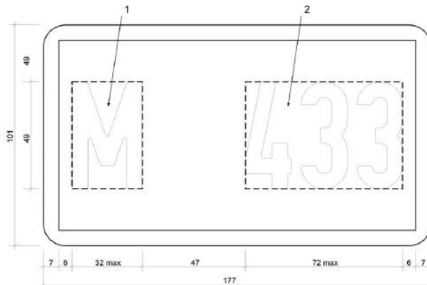
Vanasõiduki ja selle haagise registreerimismärgi mõõdud ja väljad.
